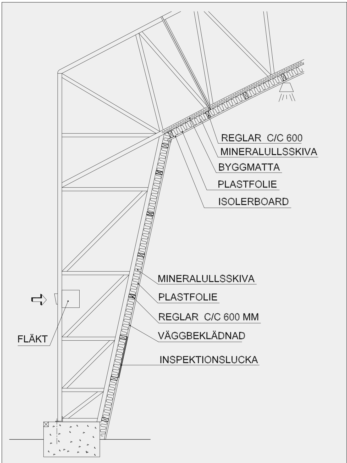
Principritning på isolering av PMH Thermohall.
